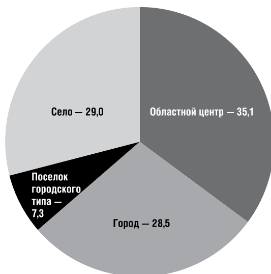
Рис. 3. Структура выборки по типу населенного пункта (%)
