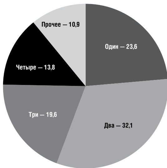
Рис. 2. Структура выборки по количеству членов семьи (%)
