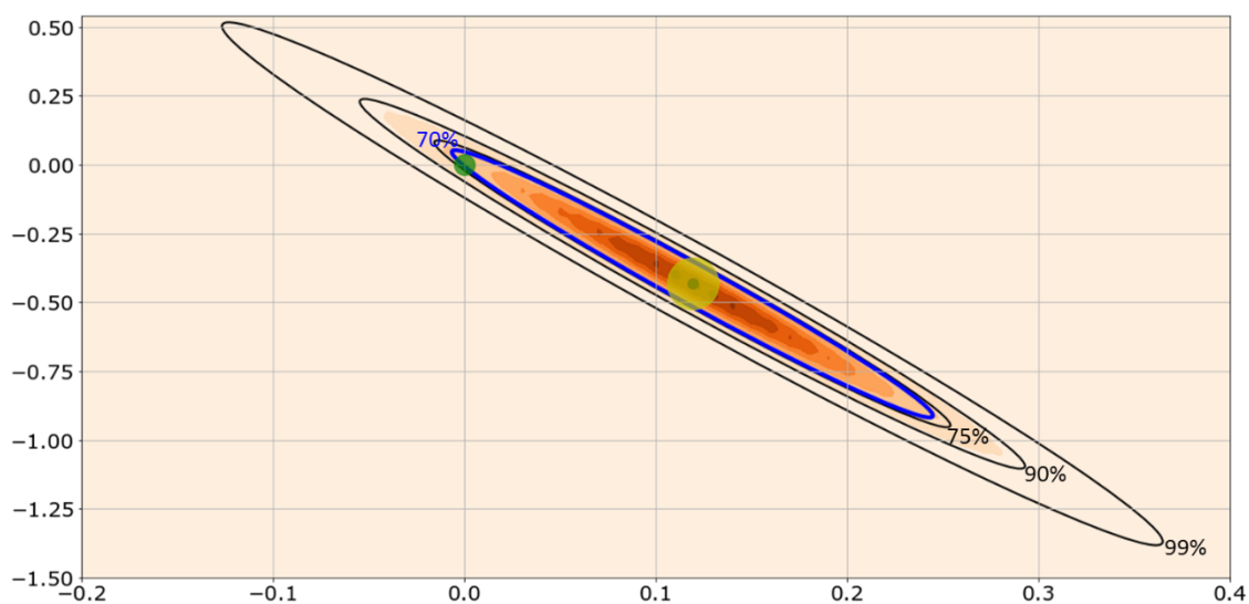
Рис. 5. Доверительные эллипсоиды для вектора параметров (\alpha', \beta')
