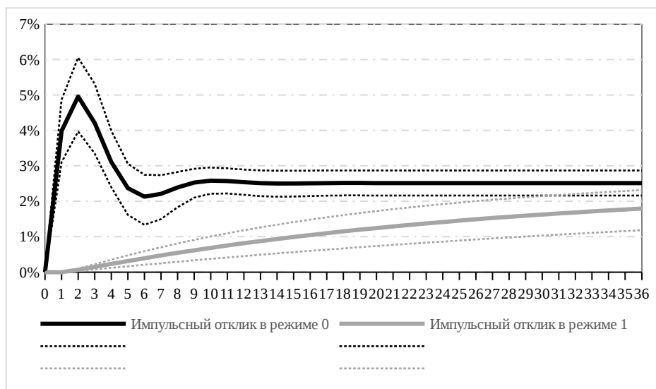
Рис. 4. Функции импульсных откликов реального обменного курса рубля на 10%-ный перманентный шок нефтяных цен
