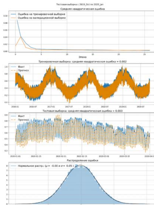
Рис. 19. Результат обучения RNN модели с тестовыми данными первого квартала 2020 года
