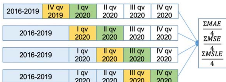
Рис. 13. Валидация выборки в процессе обучения нейронной сети
