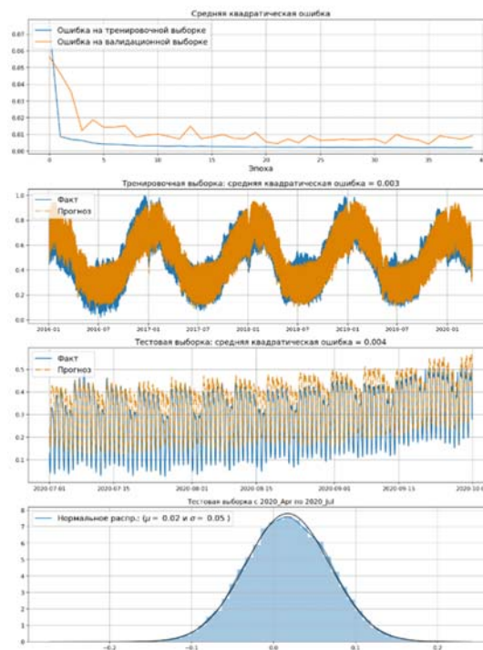
Рис. 17. Результат обучения CNN-RNN модели с тестовыми данными третьего квартала 2020 года
