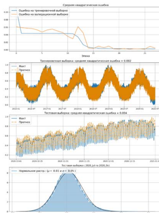
Рис. 18. Результат обучения CNN-RNN модели с тестовыми данными четвертого квартала 2020 года
