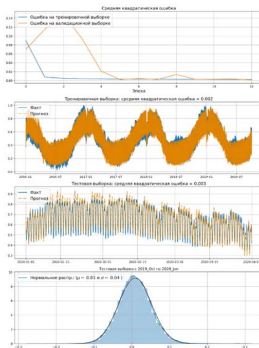
Рис. 14. Результат обучения CNN-RNN модели с тестовыми данными первого квартала 2020 года
