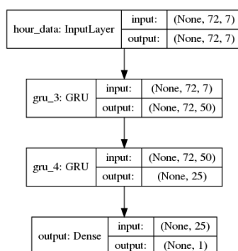
Рис. 12. Архитектура рекуррентной нейронной сети, используемой в качестве альтернативной модели
