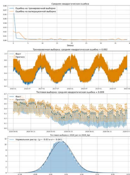
Рис. 16. Результат обучения CNN-RNN модели с тестовыми данными второго квартала
