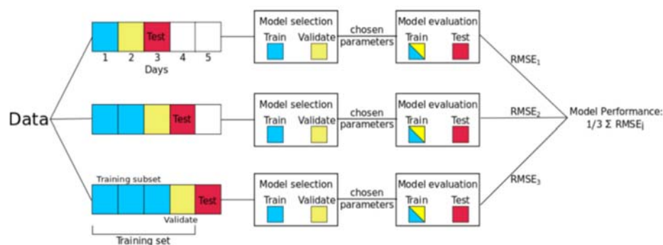
Рис. 9. Подход к кросс-валидации временных рядов
