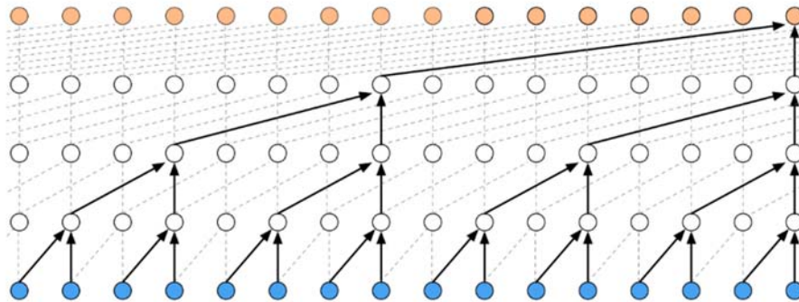
Рис. 5. Визуализация принципа работы причинной сверточной сети
