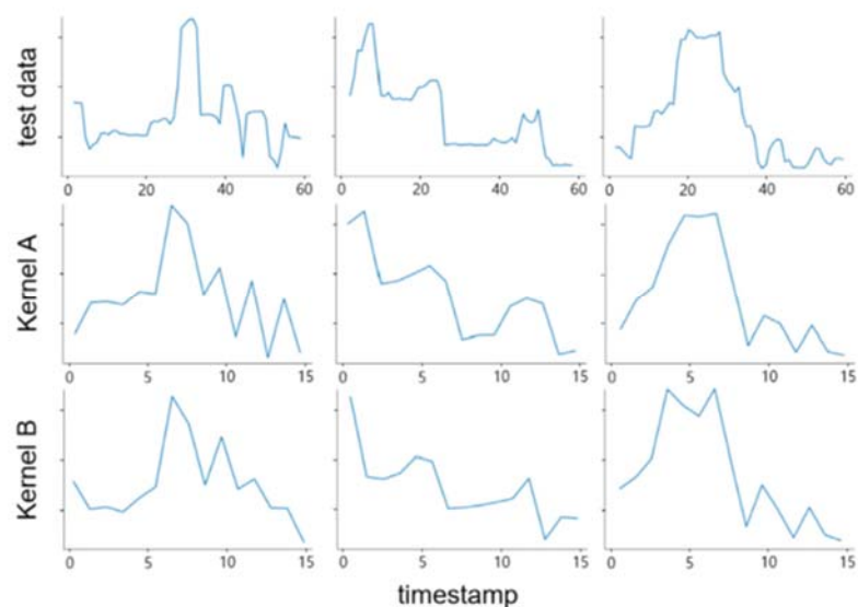
Рис. 2. Визуализация работы сверточных слоев нейронной сети
