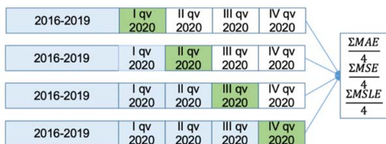
Рис. 23. Принцип валидации данных для авторегрессионной модели.
