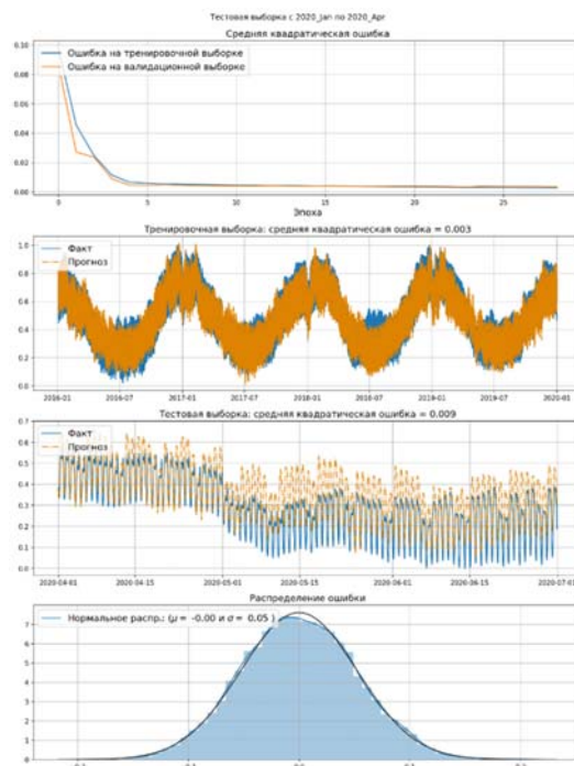
Рис. 20. Результат обучения RNN модели с тестовыми данными второго квартала 2020 года
